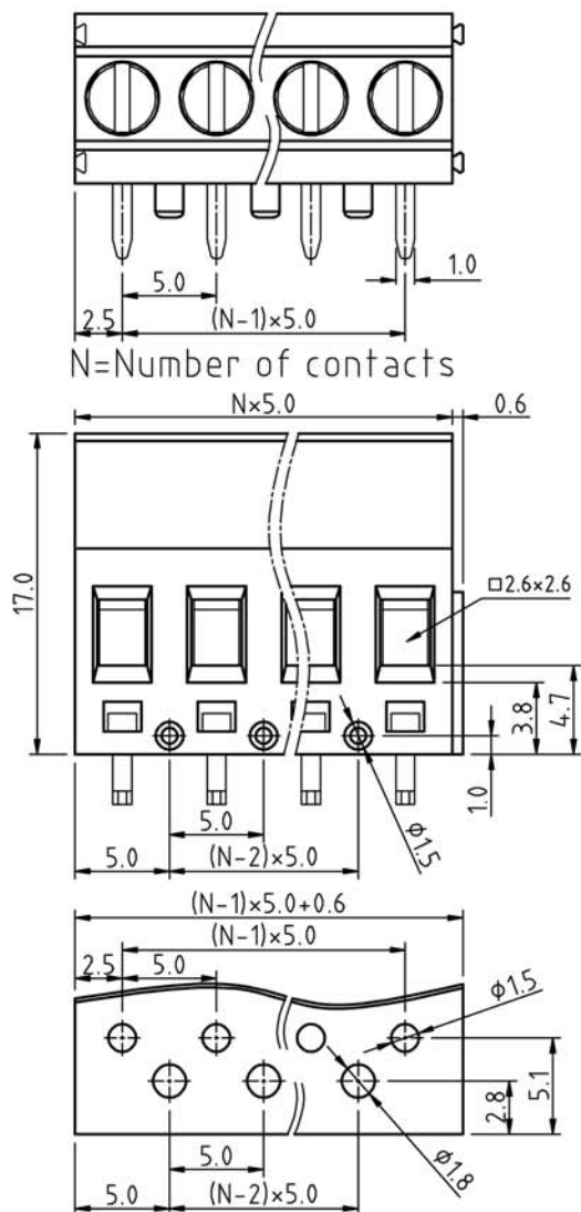
P.C.B. LAYOUT
